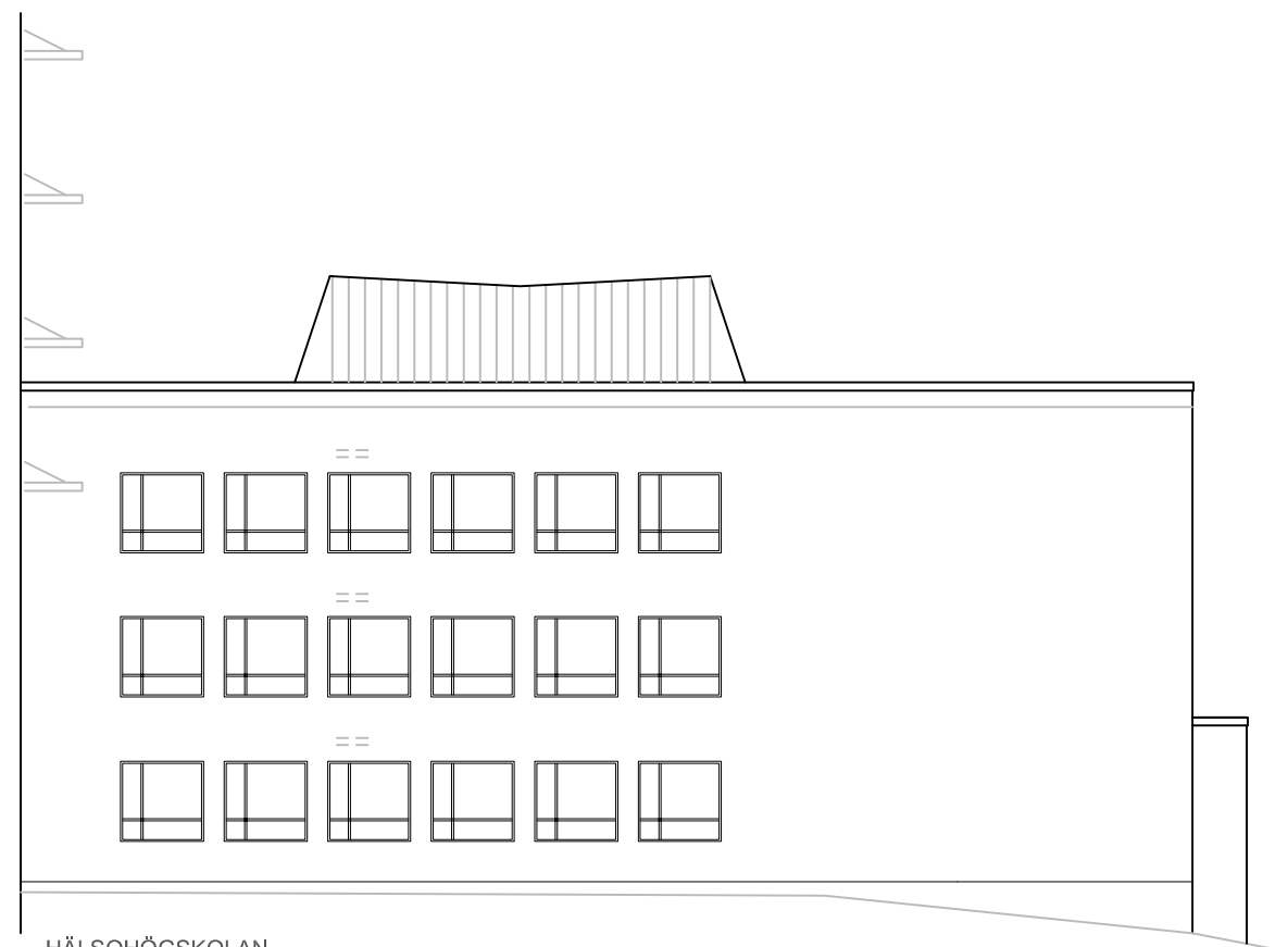
HÄLSOHÖGSKOLAN HUS D FASAD MOT VÄSTER
