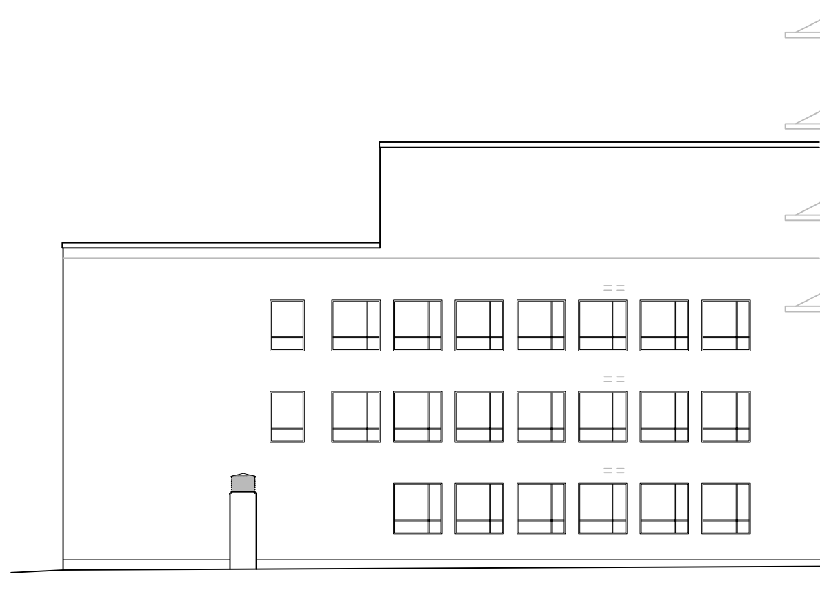
HÄLSOHÖGSKOLAN, HUS C FASAD MOT ÖSTER
